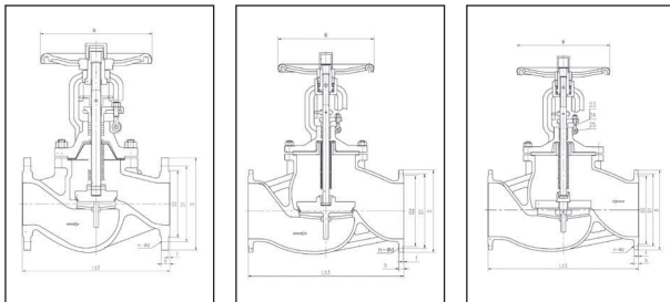
DN150
